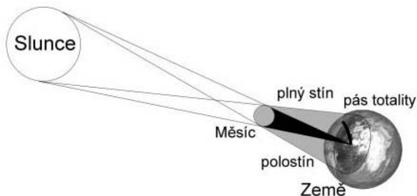
Schéma úplného zatmění Slunce
